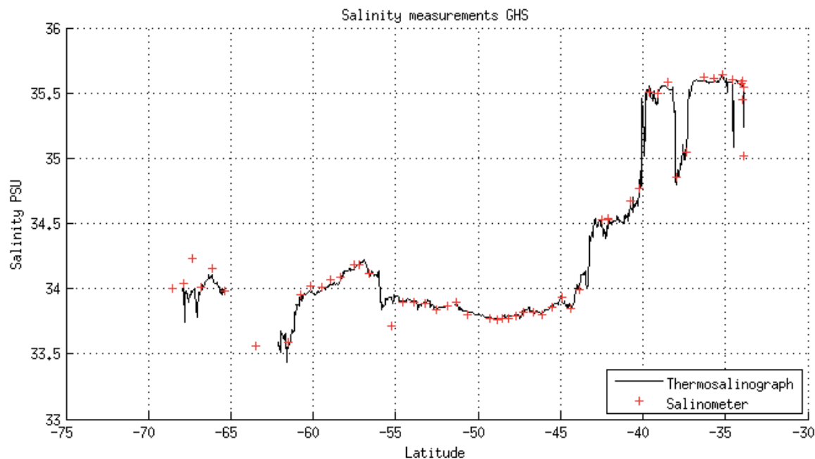
Fig. 7 : Confronto tra la salinità misurata dal TSG e quella ricavati dai campioni prelevati in situ e analizzati tramite salinometro Portasal.
