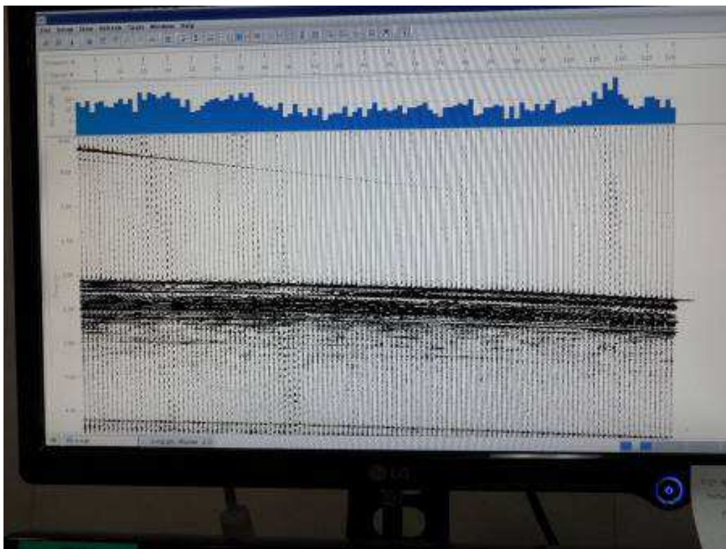
Fig. 6 – Esempio di shot gather . E' possibile notare la presenza di riflessioni sul dato raw senza applicazione di alcun guadagno di riflessioni a circa 3.450 s twt corrispondenti ad interfacce sismiche poste a profondità di circa 1200 – 1600 m al di sotto del fondo mare (circa 1500 m).
