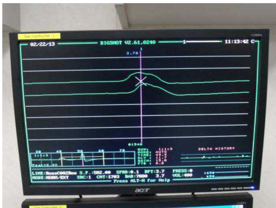
Fig. 8 – Esempio di controllo della sincronizzazione dei cannoni con il software Big Shot. Il cannone n. 3 e n. 4 risultano funzionanti e sincronizzati.
