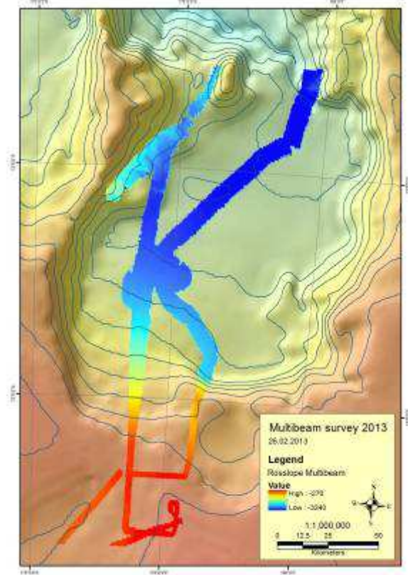
Fig. 4 – Survey MB
