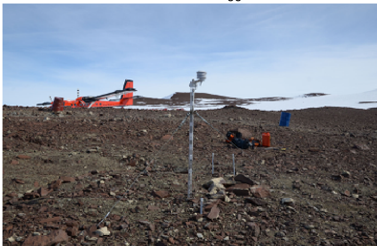
Fig. 2 - Mount Jackman: stazione monitoraggio del regime termico dei cunei di ghiaccio e ubicazione del punto di rifornimento.
