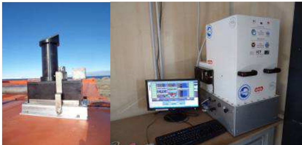
Fig. 3 - (SX) VELOD - Vertical L ooking D evice fissato sul tetto del Container denominato PAT. Si nota il raccordo tra VELOD e tetto per l'ingresso della fibra ottica realizzato con un tubo rigido a protezione della fibra stessa. (DX) GASCOD-NG1/SPATRAM-MZS installato all'interno del PAT.
