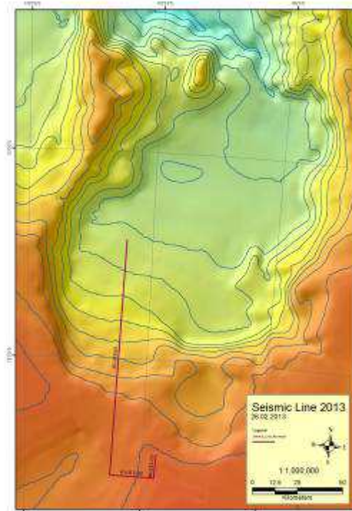
Fig. 5 – Rilievo sismico
