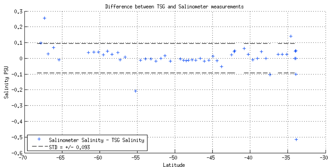
Fig. 8: Differenza in salinità tra i valori misurati dal TSG e quelli ricavati dai campioni prelevati in situ e analizzati tramite salinometro Portasal.
