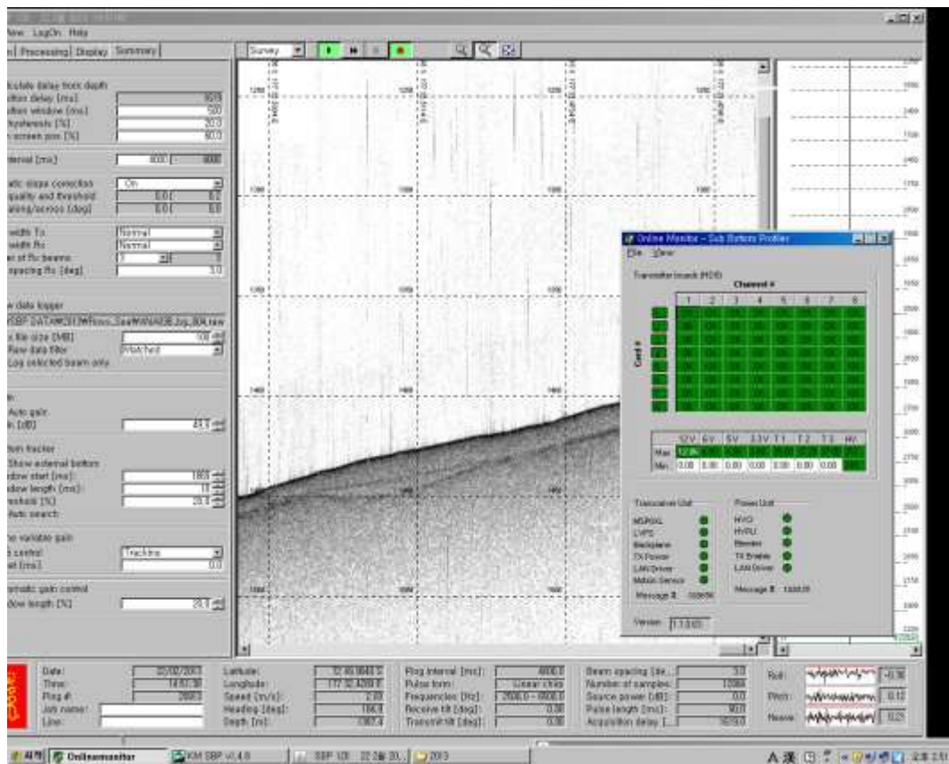
Fig. 11 – Sub bottom profile: controllo di qualità sul funzionamento e qualità dato.
