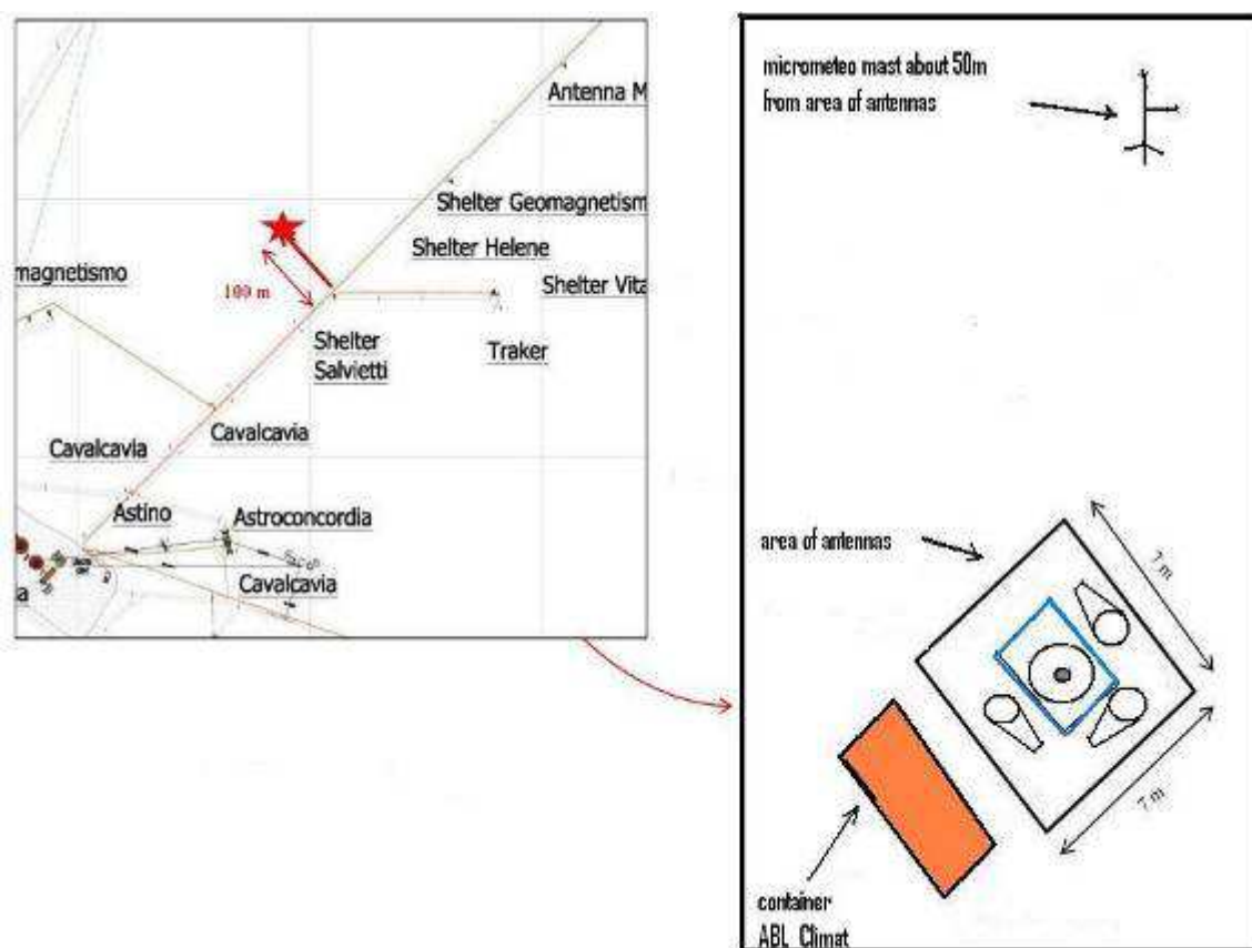
Fig. 3. Posizione in campo dell' SLM-SODAR (stella rossa - pannello di sinistra), disposizione delle antenne campo rispetto allo shelter (pannello di destra).
