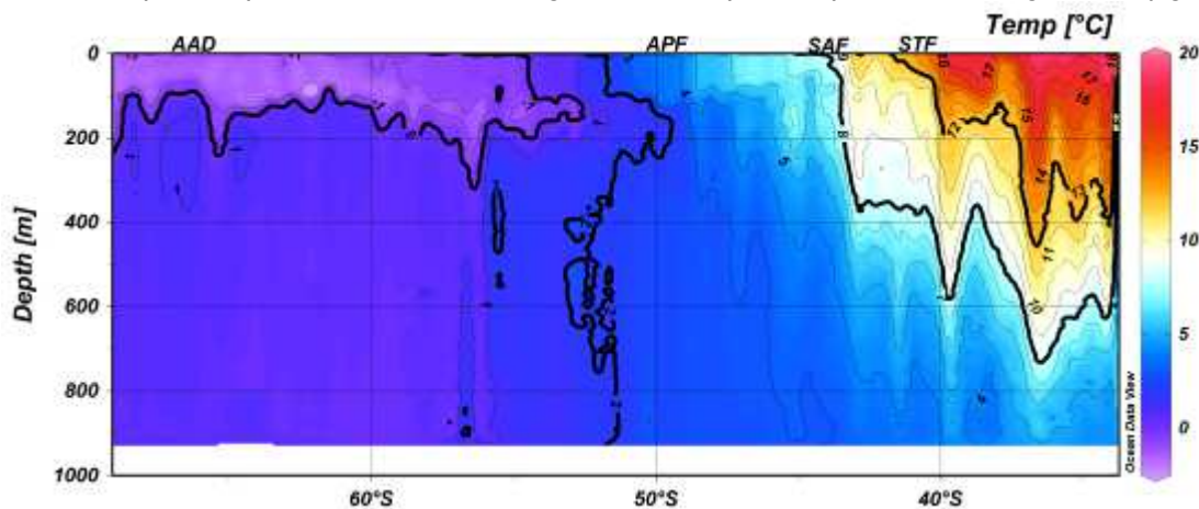
Figura 4 : Sezione di temperatura relativa al transetto Città del Capo – Antartide, 6-15 dicembre 2012.
