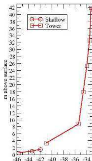
Profil de température mesuré le 5 Février 2013 à 3:30 le matin. Le profil de la tour est complété par les données de la station de profilage de surface re-déployée à proximité du shelter « neige ».
