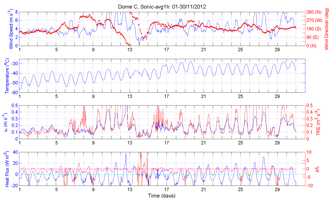
Fig. 5. Serie temporale delle misurazioni ottenute dall' anemometro sonico: velocità del vento, direzione, temperature sonica, velocità di attrito, flusso di calore sensibile per il periodo 01 – 30 novembre 2012.
