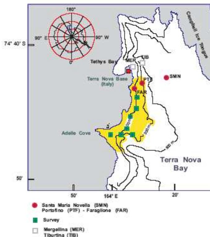
Fig.1: Area marina protetta e stazioni storiche
