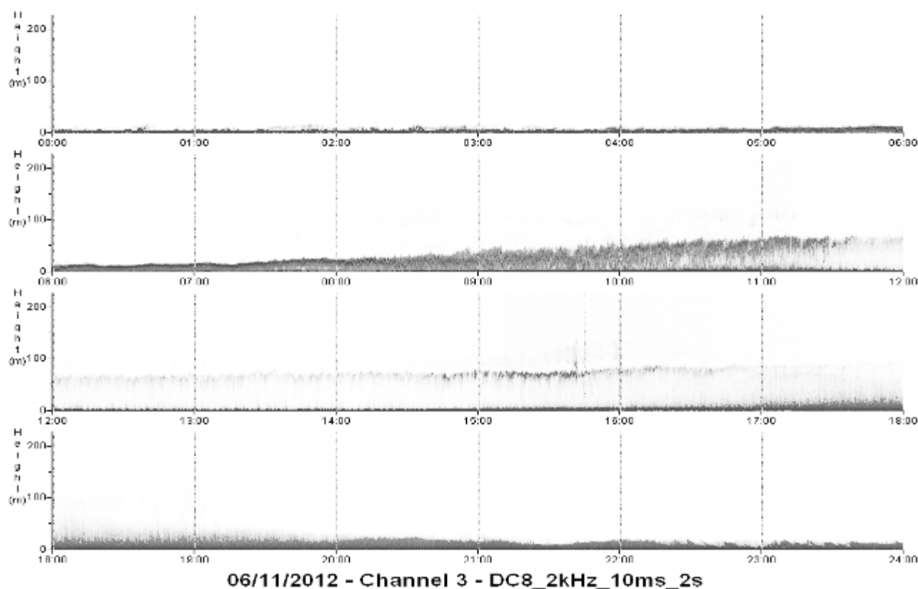
Fig. 6. Evoluzione temporale dello strato limite atmosferico come vista dal SLM-SODAR (06 novembre 2012).
