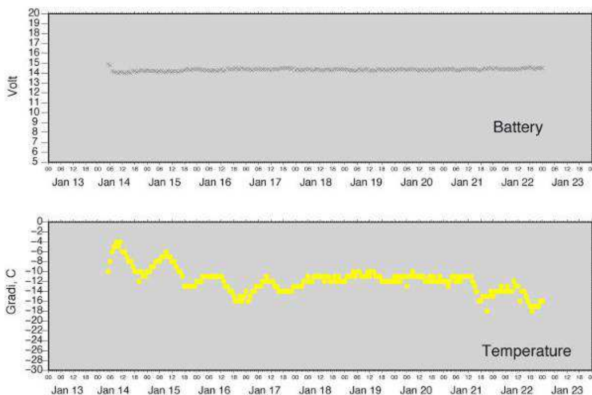
Fig. 1: Funzionamento della stazione TALOS DOME. In alto, l'andamento del voltaggio, in basso, l'andamento della temperatura all'interno della cassa
