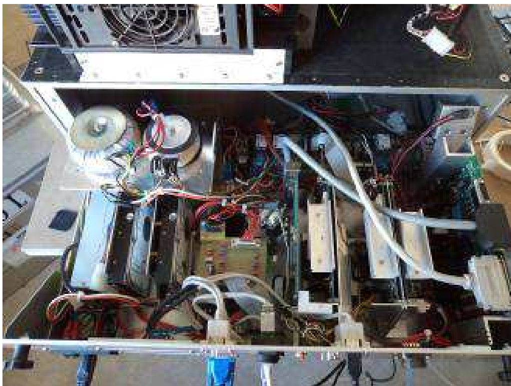
Fig. 4 - Unità elettronica di controllo - Electronic Control Unit - ECU dello spettrometro .
