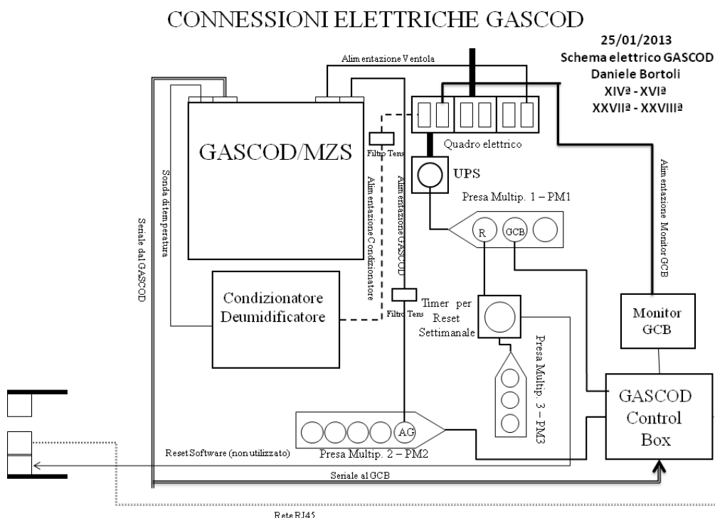
Fig. 1 - Schema delle connessioni elettriche GASCOD
