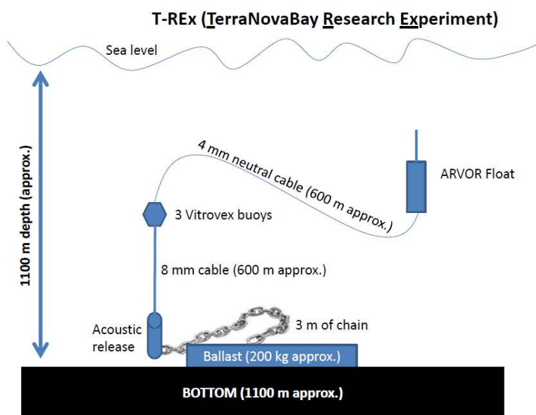
Fig. 3 - Schema ancoraggio ARGO float
