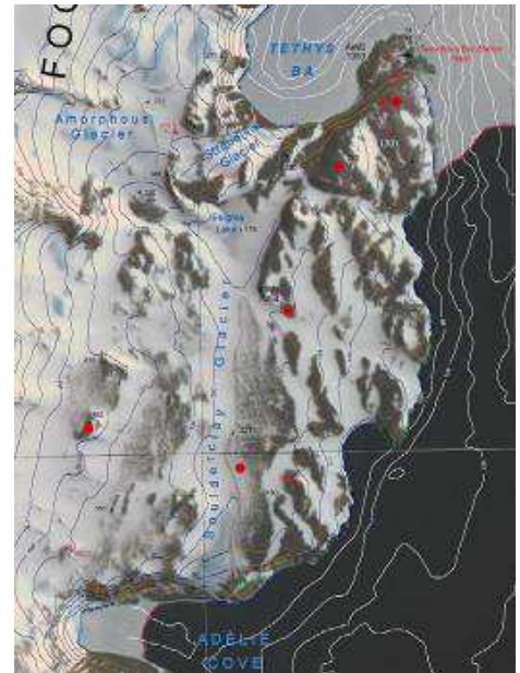
Fig. 2 Posizione delle 5 AWS e del sodar nell'aerea di Terra Nova Bay
