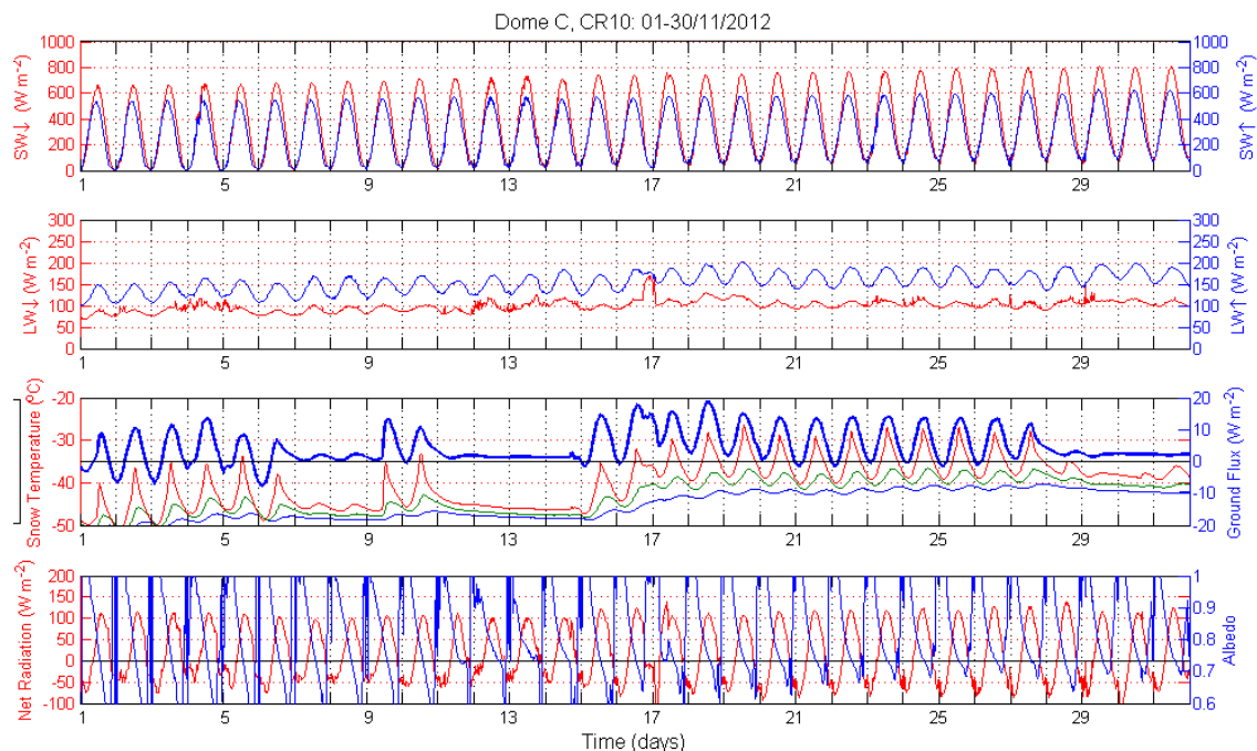
Fig. 4. Serie temporale della radiazione ad onda corta proveniente dall' atmosfera (SWDown), riflessa dal terreno (SWUp), trasmessa dall' atmosfera (LWdown), emessa dal terreno (LWup), dei sensori di temperatura posti nella neve a 0 (linea nera), 5 (linea rossa), 15 (linea verde), 30 cm (linea azzurra), il flusso di calore nel terreno (linea azzurra spessa), radiazione netta, per il periodo 01 - 30 novembre 2012.
