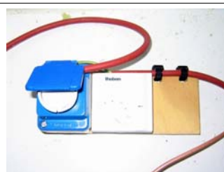
Thermostat niche 1 (la lampe est à gauche).
