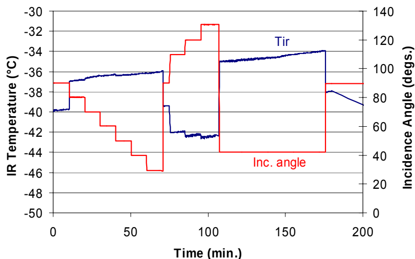
Fig. 2.9 - Esempio di dati all'infrarosso raccolti durante un ciclo di misura.
