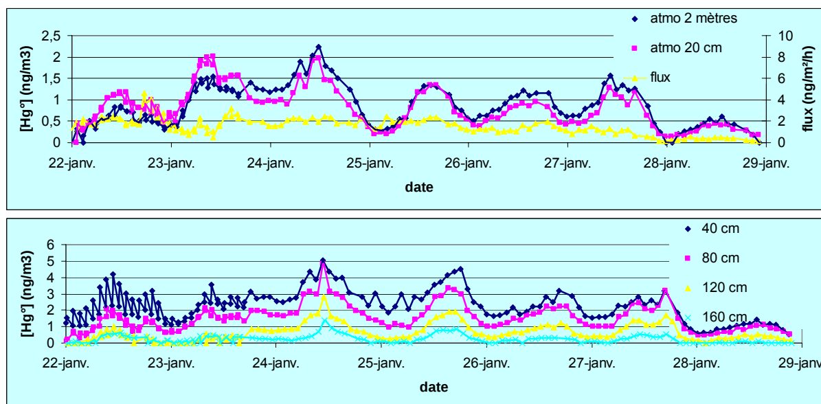
Concentrations en Hg^0 dans l'atmosphère, à 20 centimètres et 2 mètres de hauteur. Flux de Hg^0 de la neige vers l'atmosphère. Concentrations en Hg^0 dans la neige (40 cm, 80 cm, 120 cm, 160 cm de profondeur)
