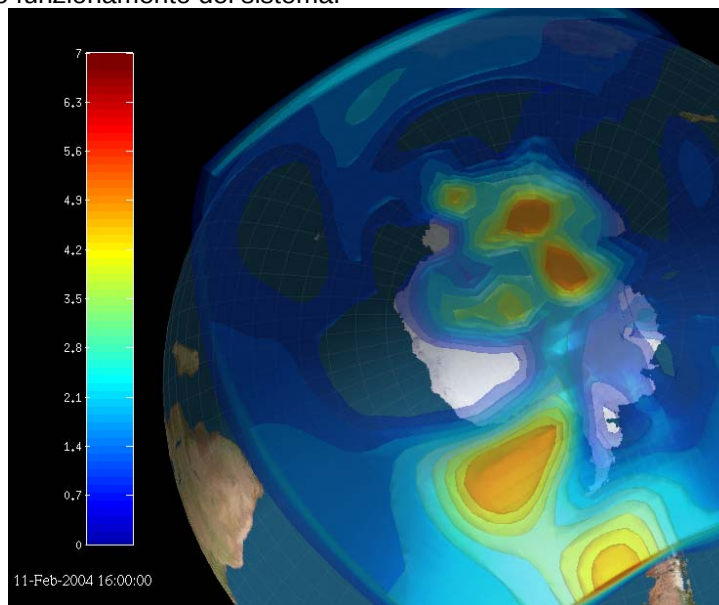
Fig. 1.5 - Concentrazione elettronica della ionosfera antartica durante un evento di scintillazione registrato a febbraio 2004: la ricostruzione è stata fatta utilizzando i dati della rete IGS (International GPS Service), i dati della comunità geodetica e quelli gestiti dalla comunità ionosferica.
